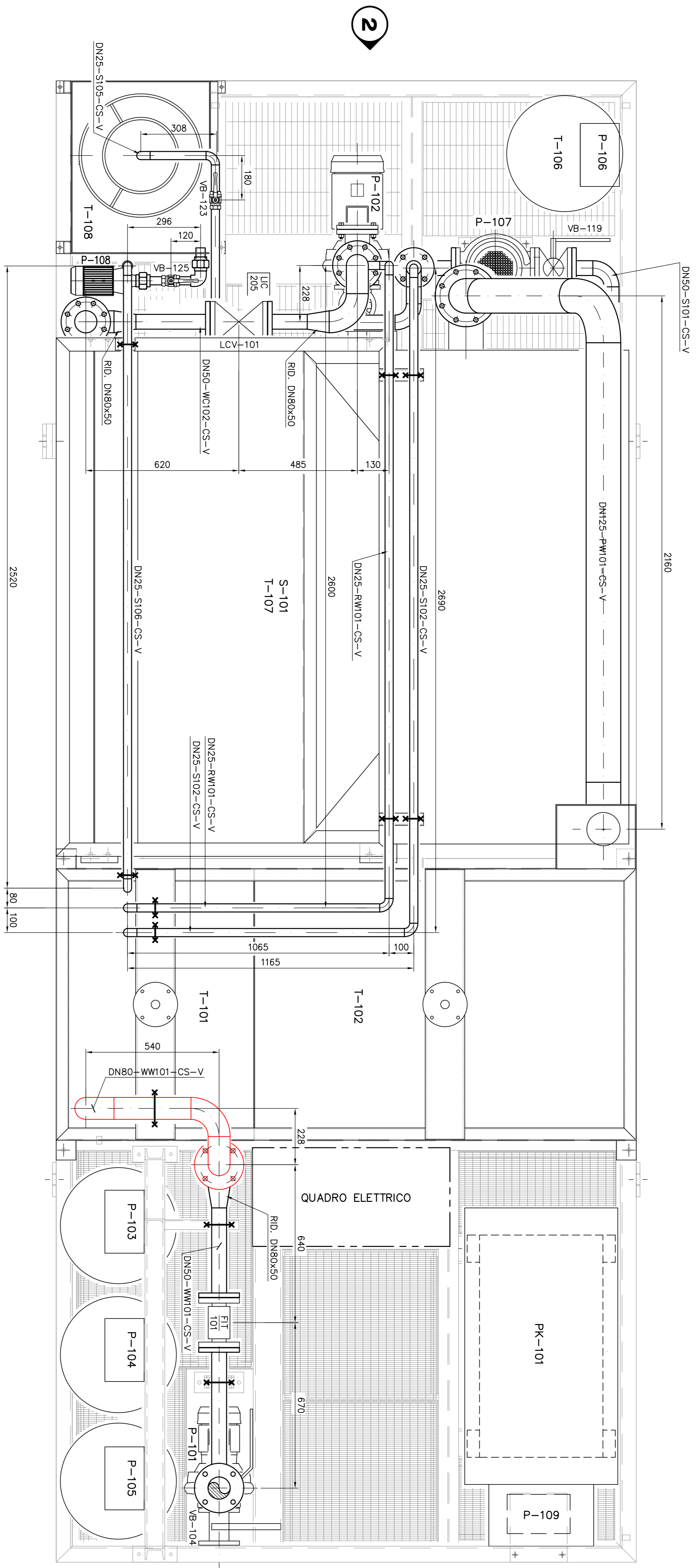
PIANTA
