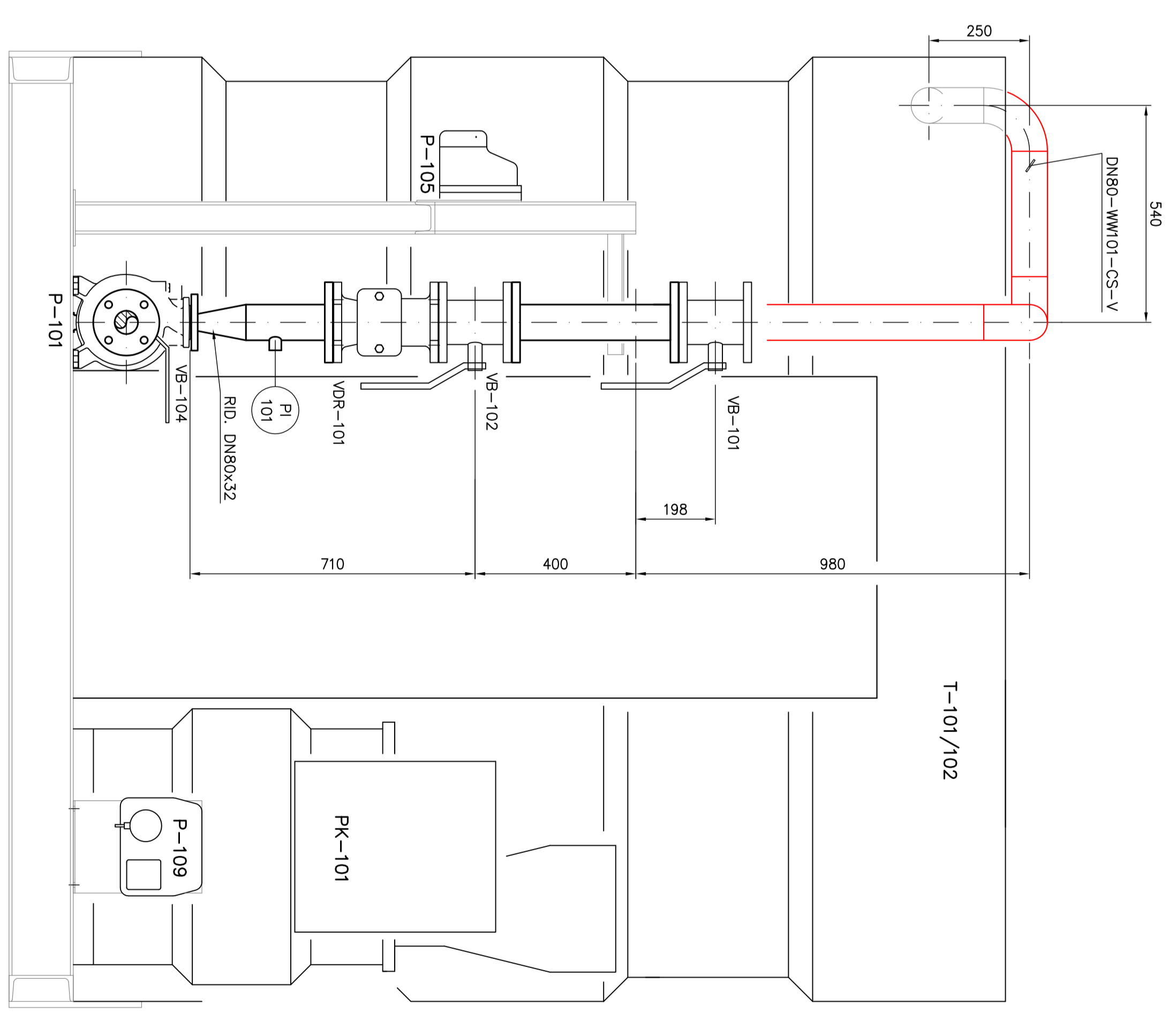
VISTA "4"
