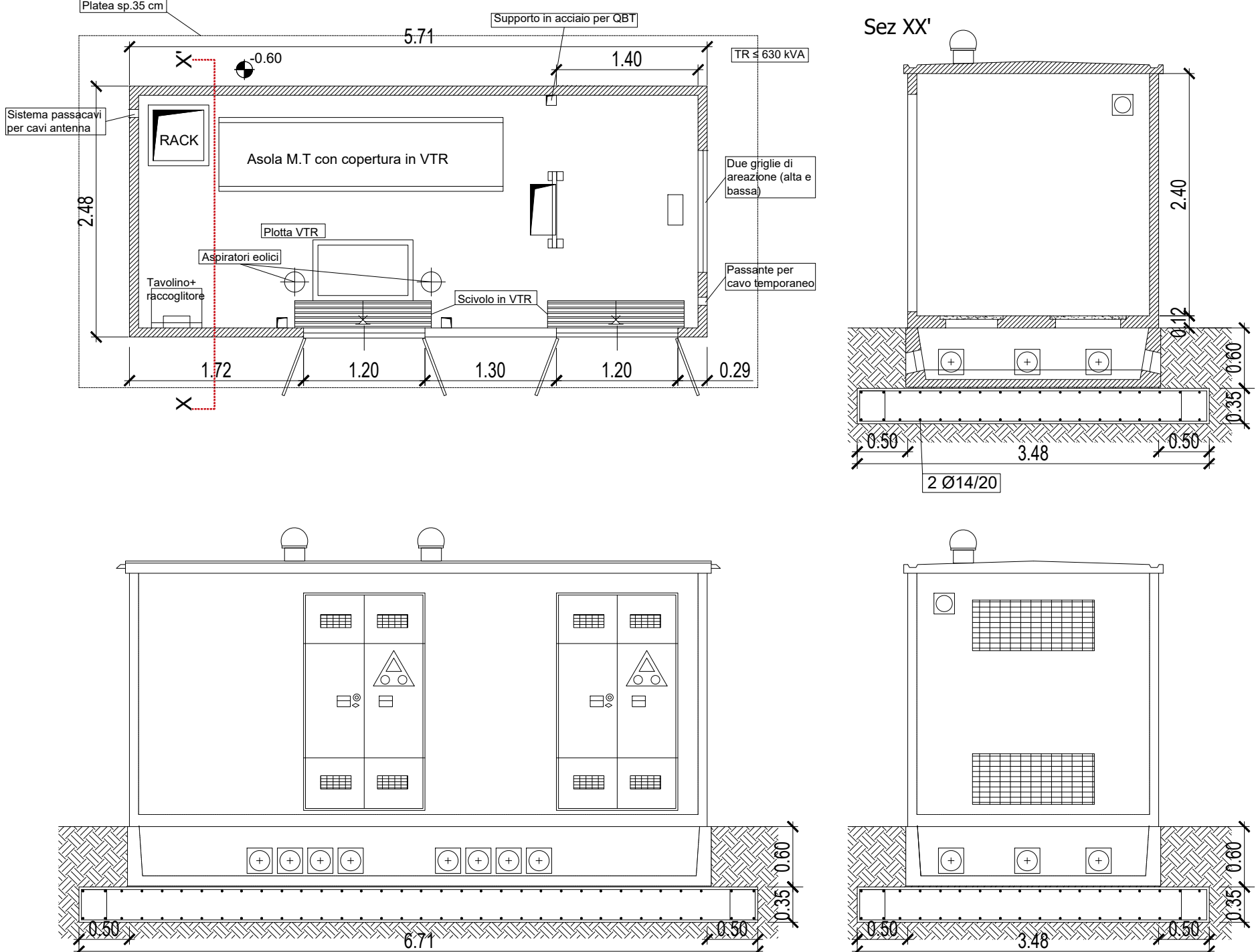
CABINA ENEL scala 1:50 Standard Box Distribuzione DG 2061/1 matricola 227280 con porte vetroresina
