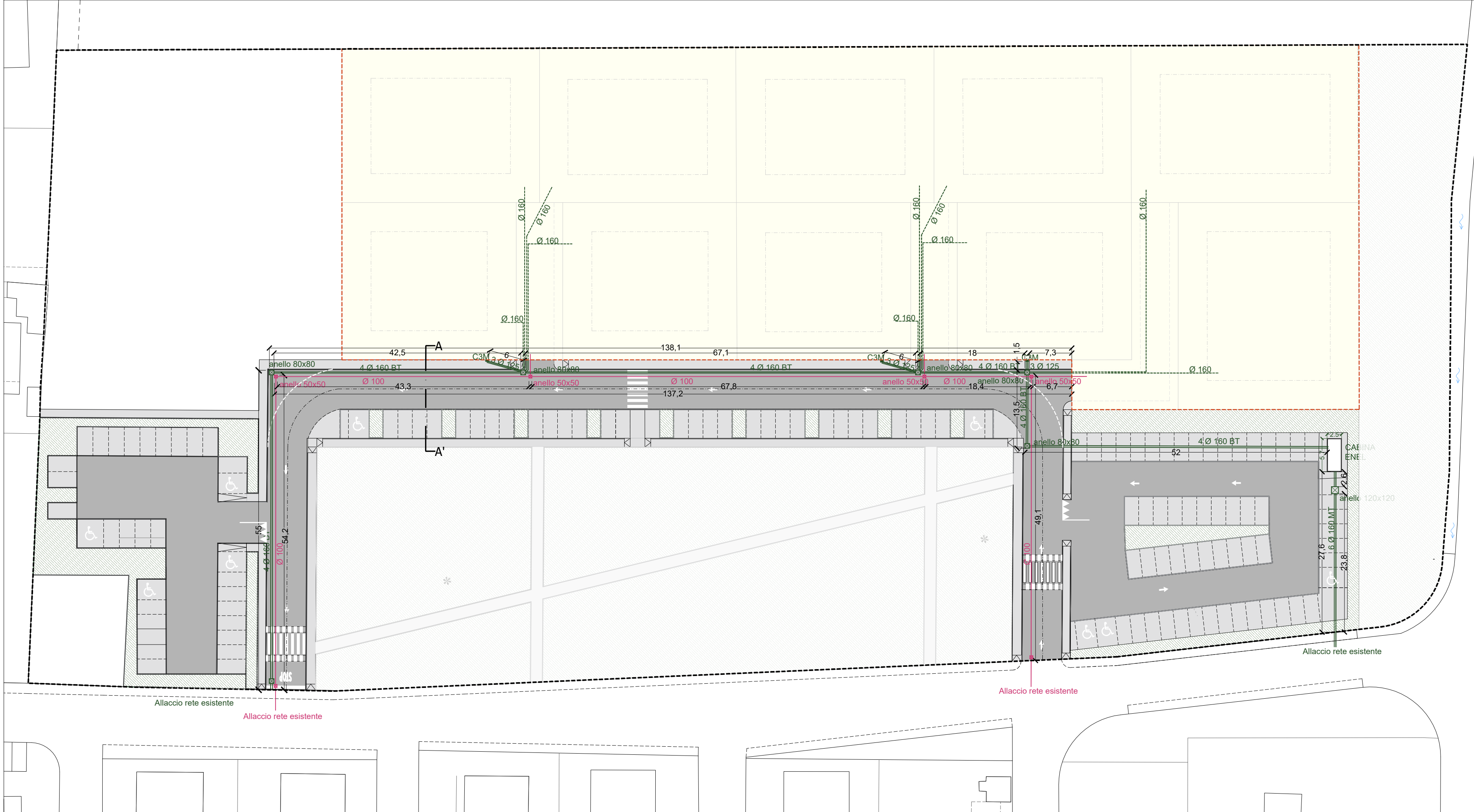
Linea Enel e Telecom scala 1:500
