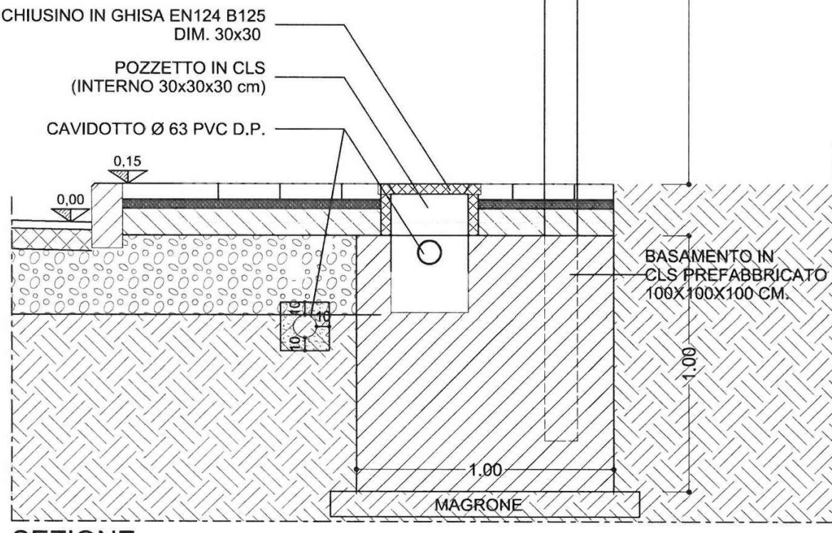
SEZIONE
