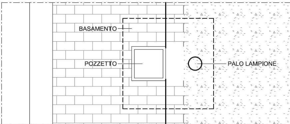
PIANTA
