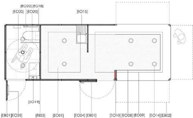
Esempio di chiosco con unità servizi igienici accessibili, da produzione a catalogo
