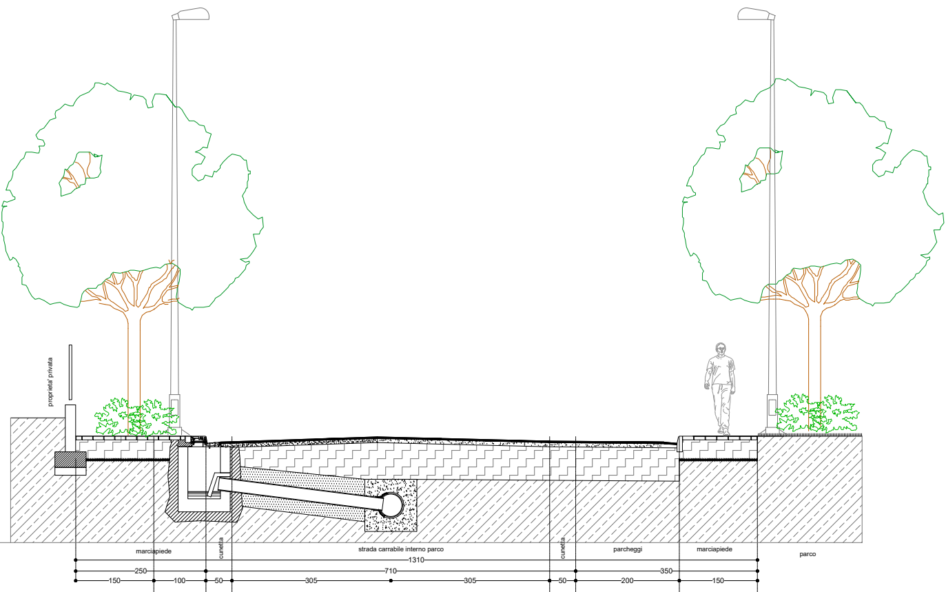
SEZ. A-A
